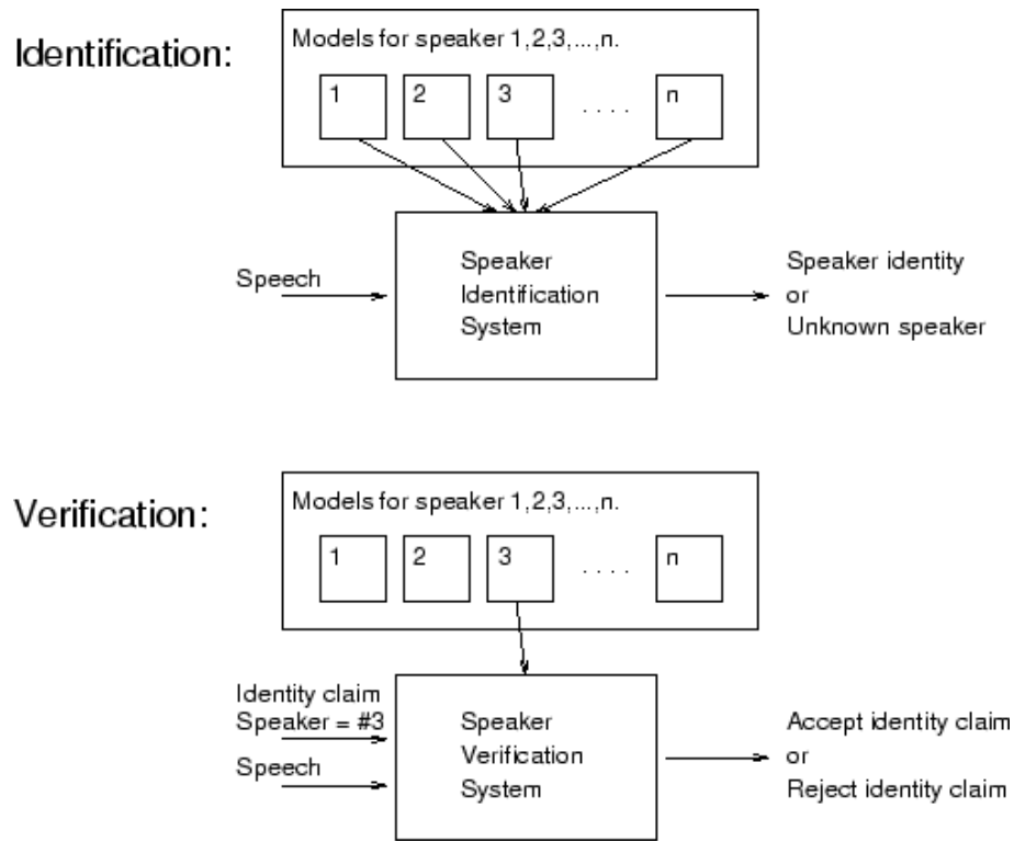
Figuur 2: Sprekerverificatie vs. sprekeridentificatie
